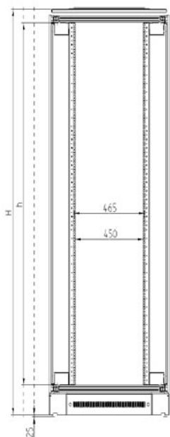
Vertiv™ Knürr® MIR2 Network Rack
